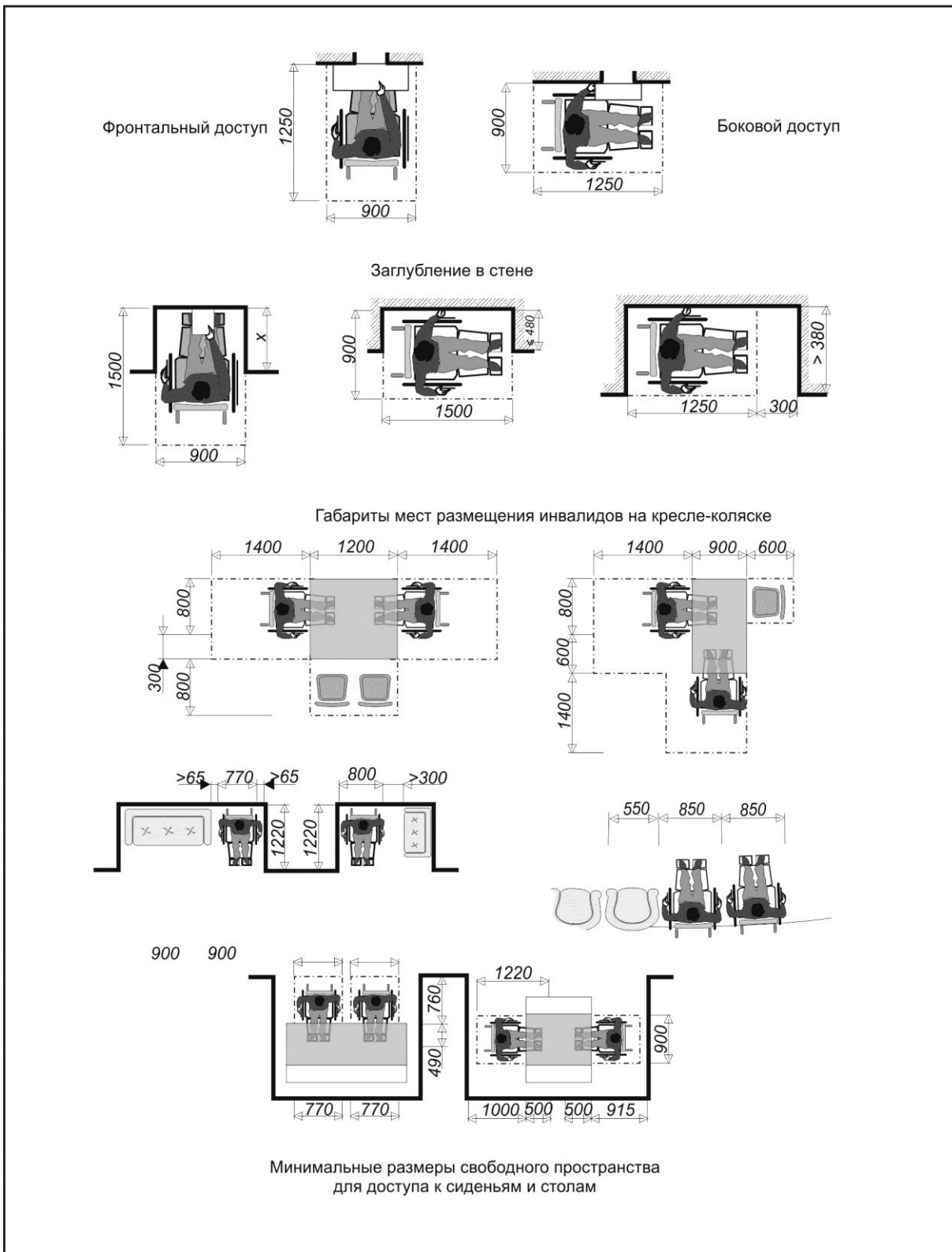
Рисунок Г.4 Габариты у мест обслуживания
