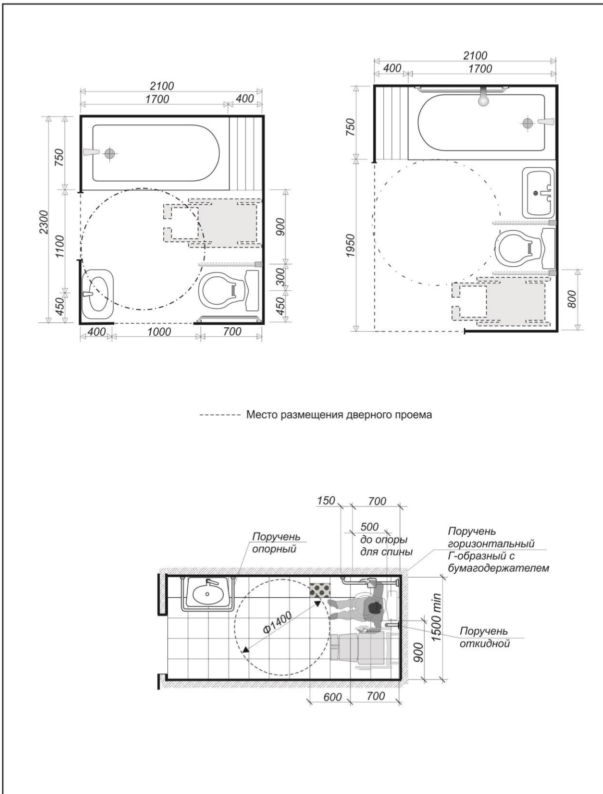
Рисунок Г.10 Совмещенный санитарный узел
