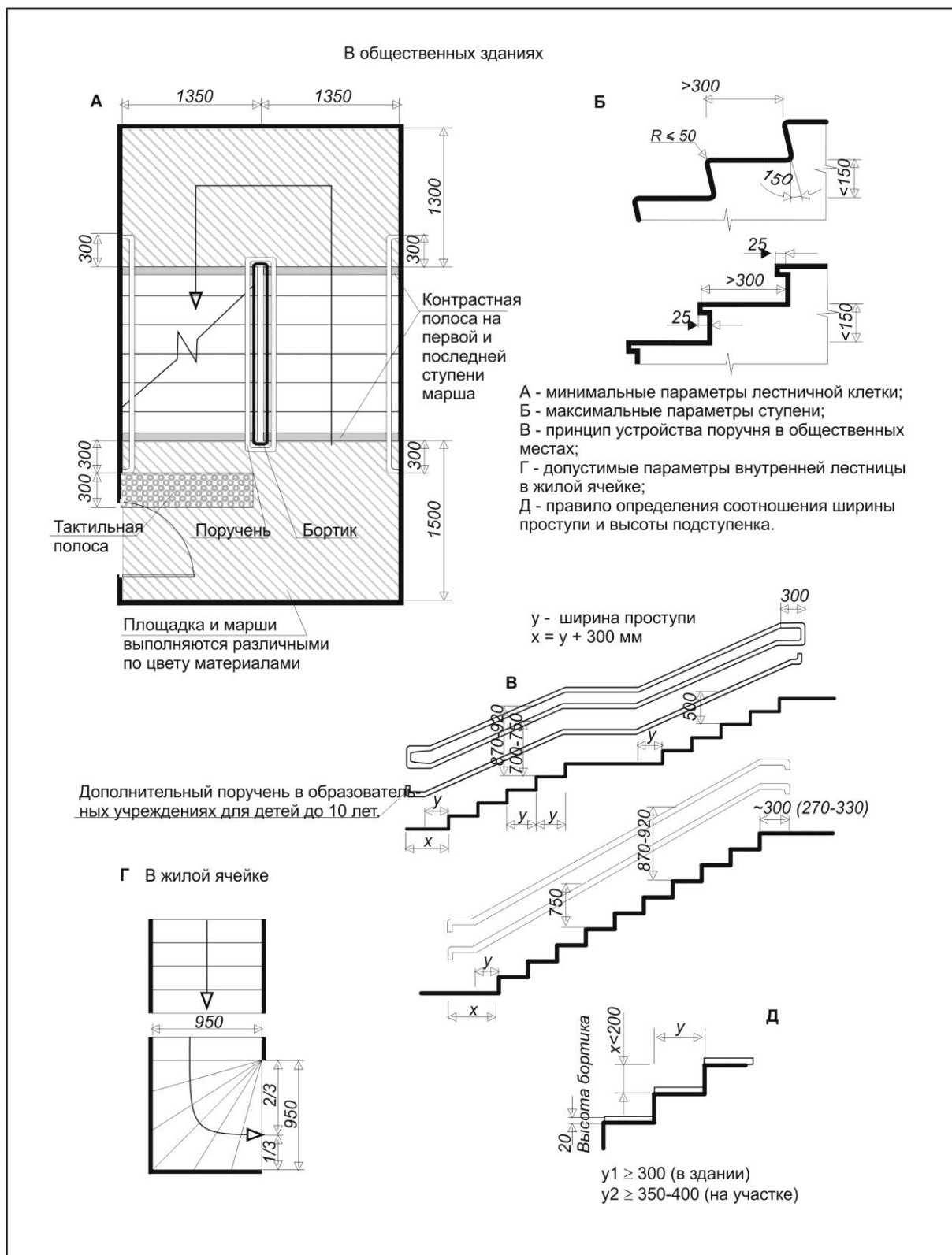
Рисунок В.18 Лестницы в общественных зданиях и в жилой ячейке
