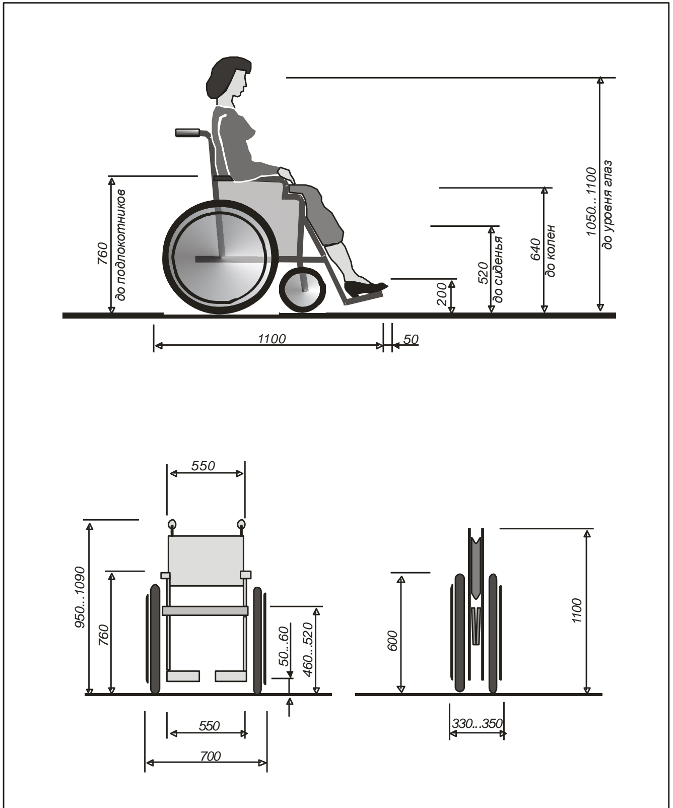
Рисунок В.1 Габариты кресла-коляски
