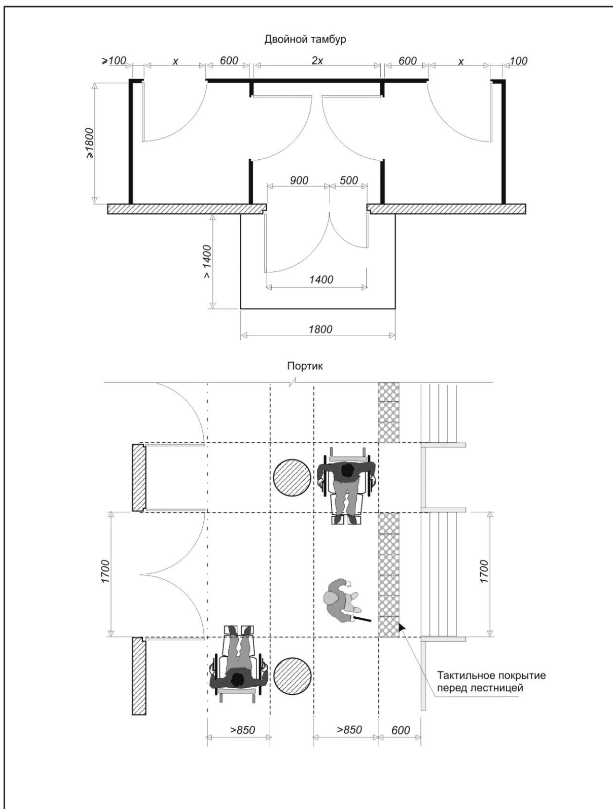
Рисунок В.16 Площадки перед тамбуром и портиком
