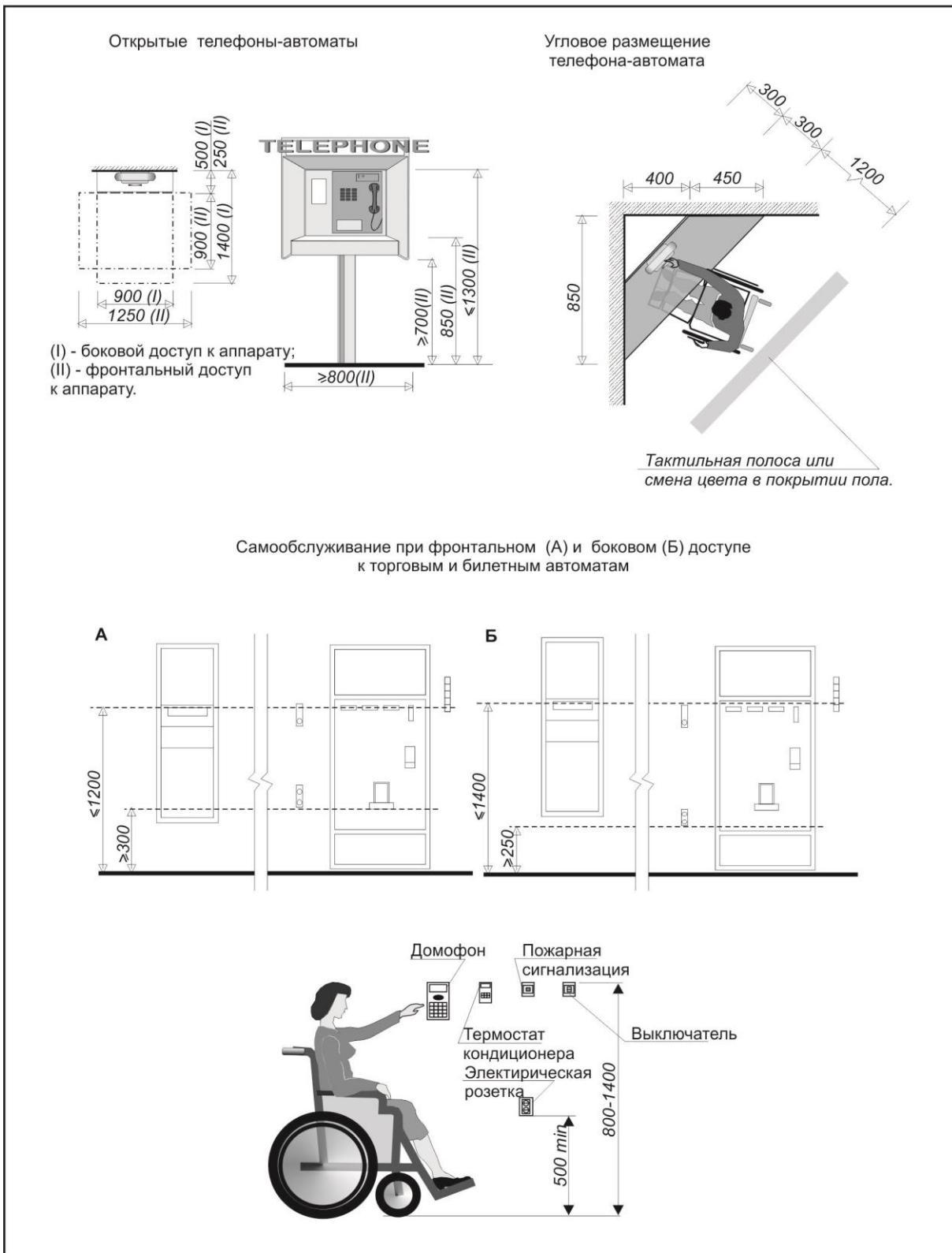
Рисунок Г.6 Досягаемость оборудования
