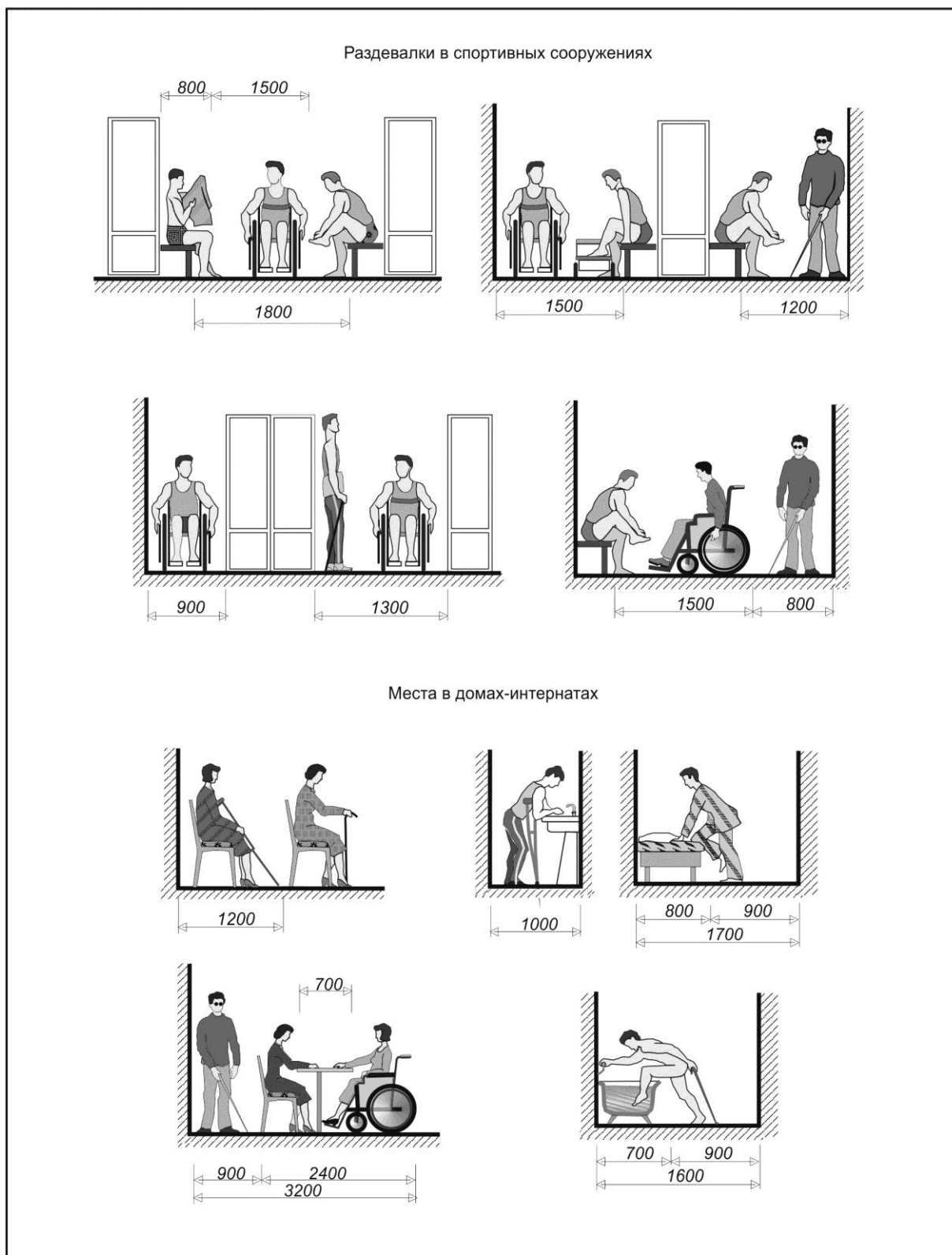
Рисунок Г.5 Параметры функциональных зон
