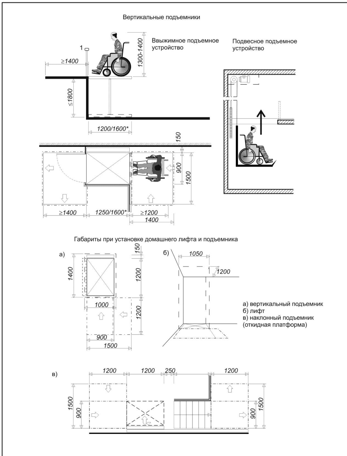
Рисунок В.26 Параметры вертикальных подъемников
