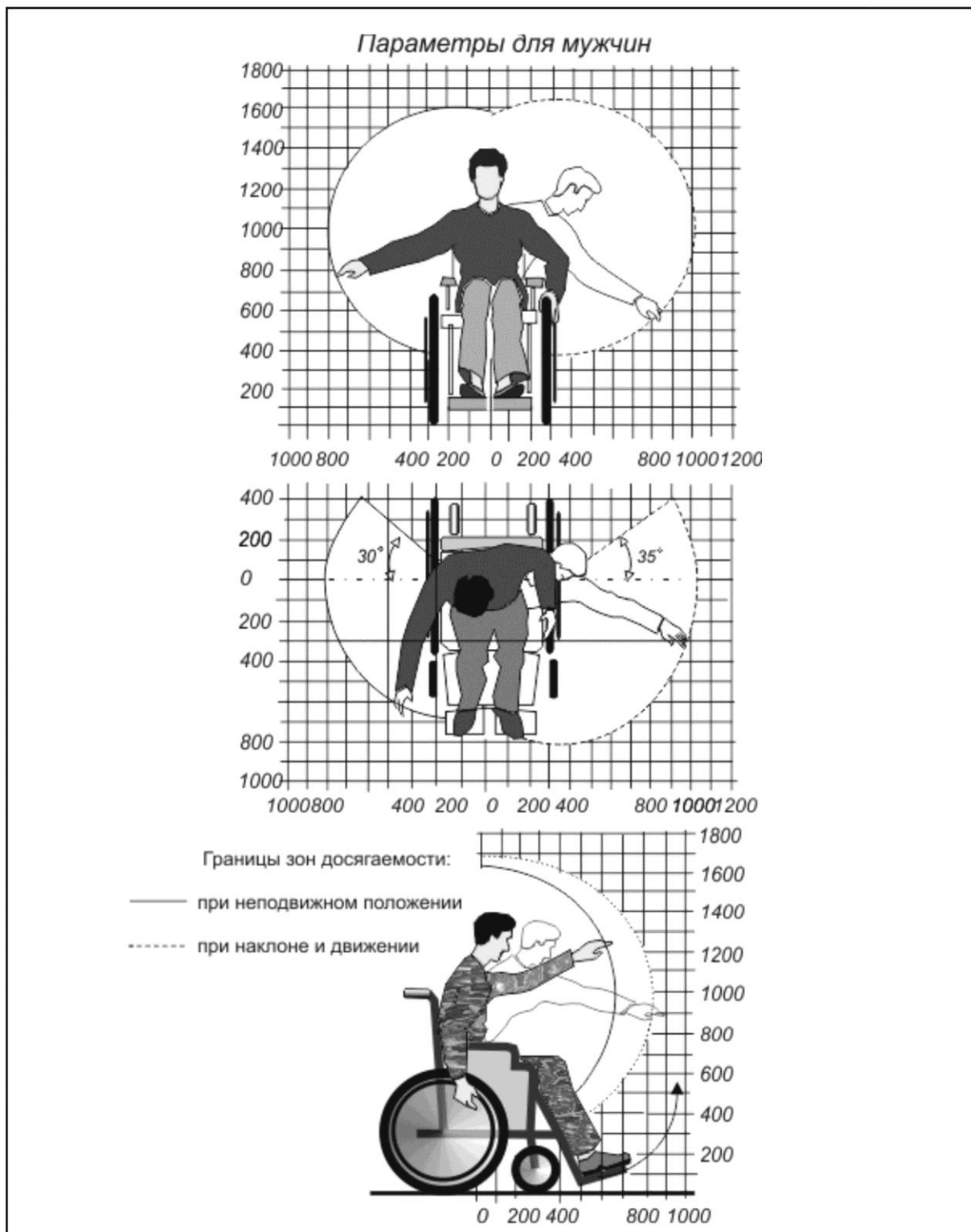
Рисунок Г.1 Зоны досягаемости инвалидов на кресле-коляске для мужчин
