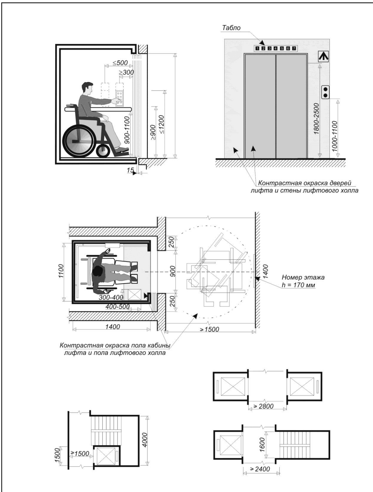
Рисунок В.24 Оборудование лифтов
