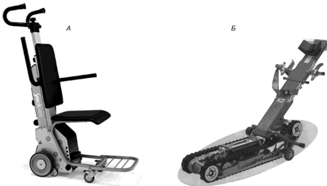
А. Колесный подъемник. Б. Гусеничный подъемник.
