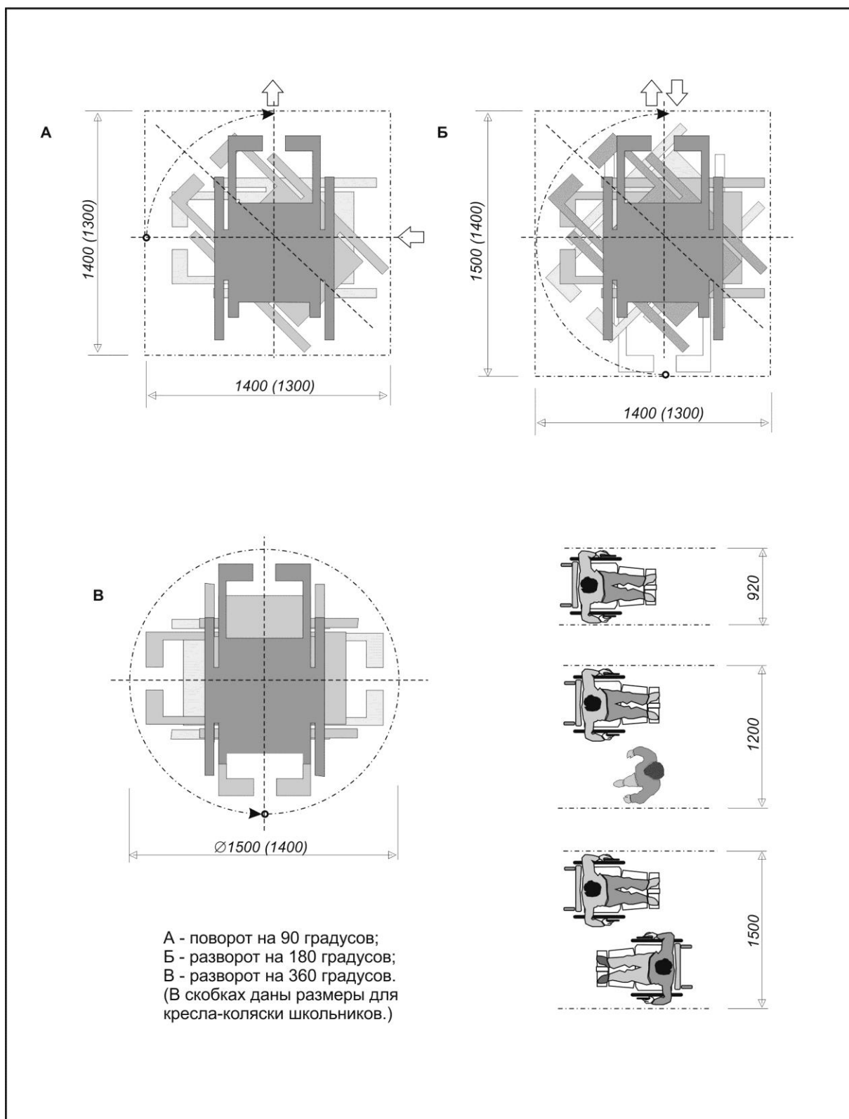
Рисунок В.3 Параметры занимаемой зоны при вращении и движении МГН на кресле-коляске
