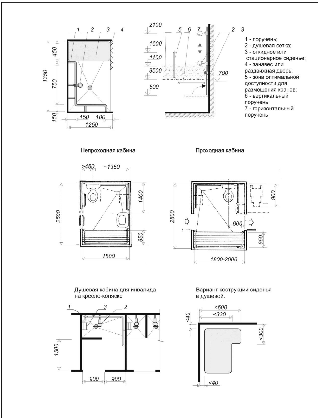
Рисунок Г.9 Габариты душевых кабин
