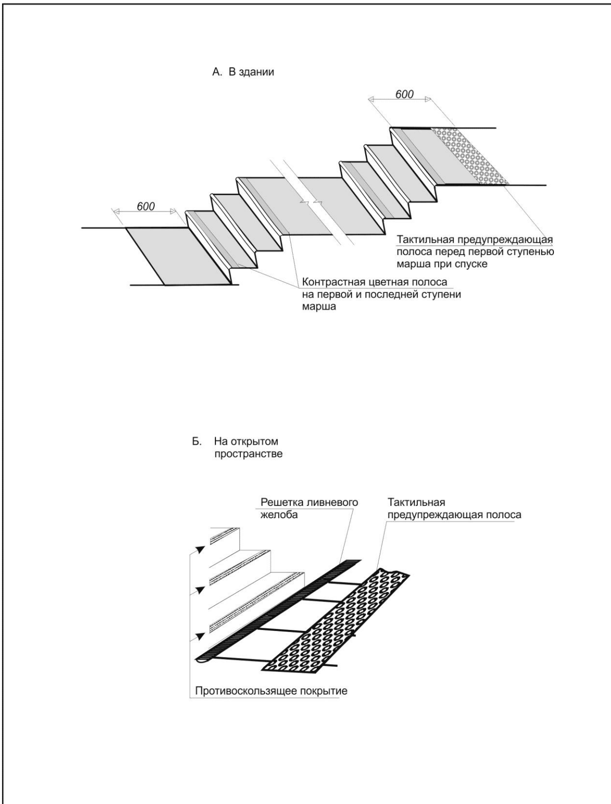
Рисунок В.19 Предупреждающие и тактильные полосы на лестницах
