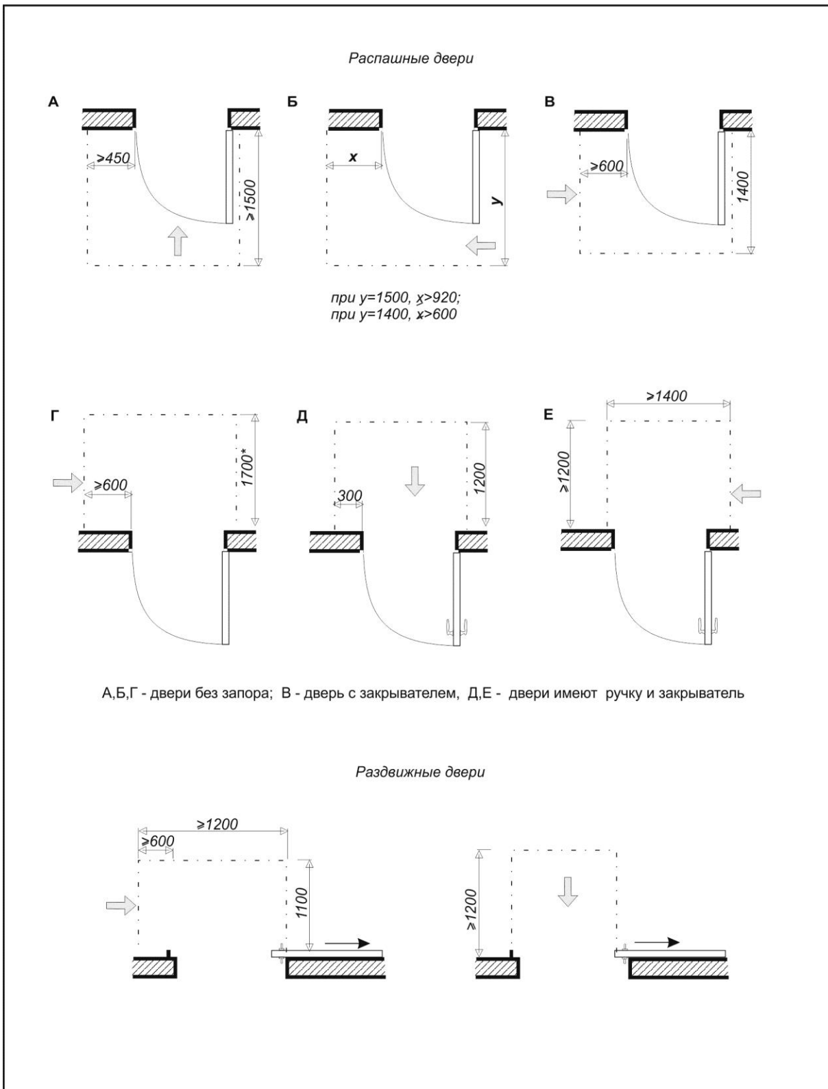
Рисунок В.13 Габариты придверных зон
