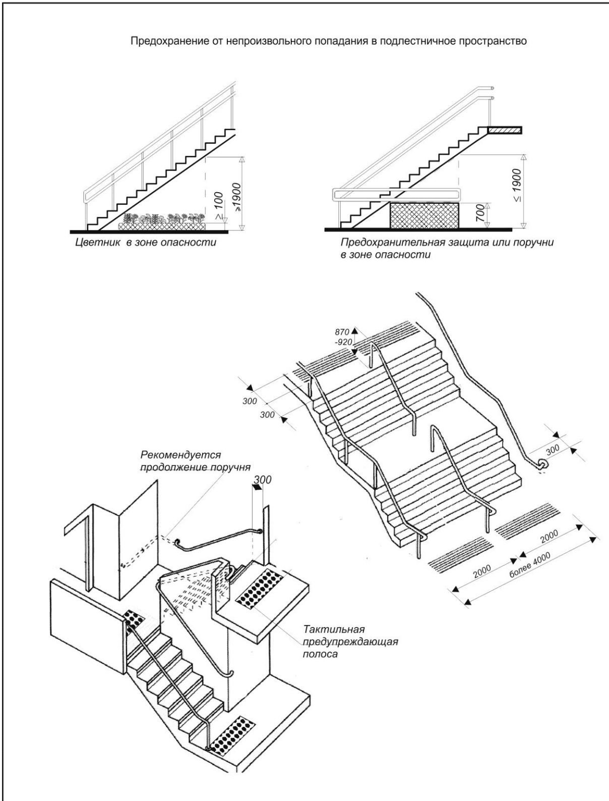
Рисунок В.17 Параметры лестниц
