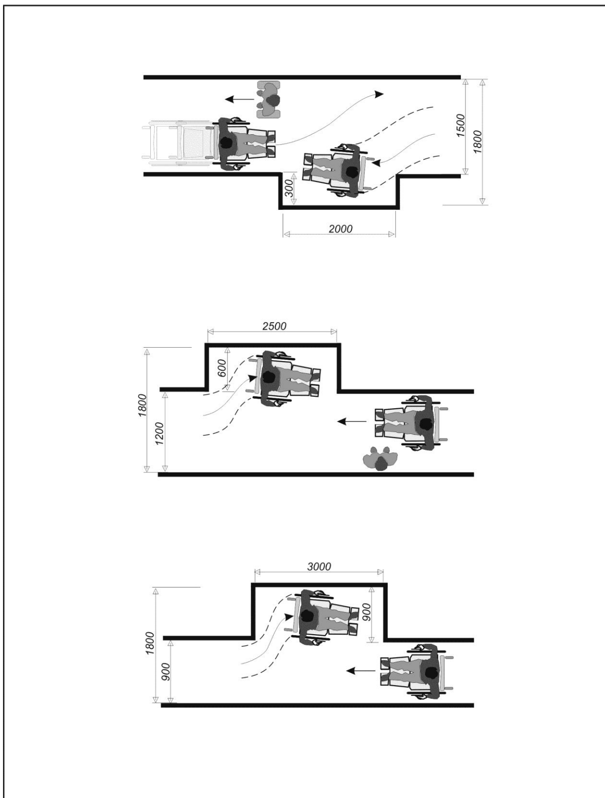
Рисунок В.8 Ниши в коридорах
