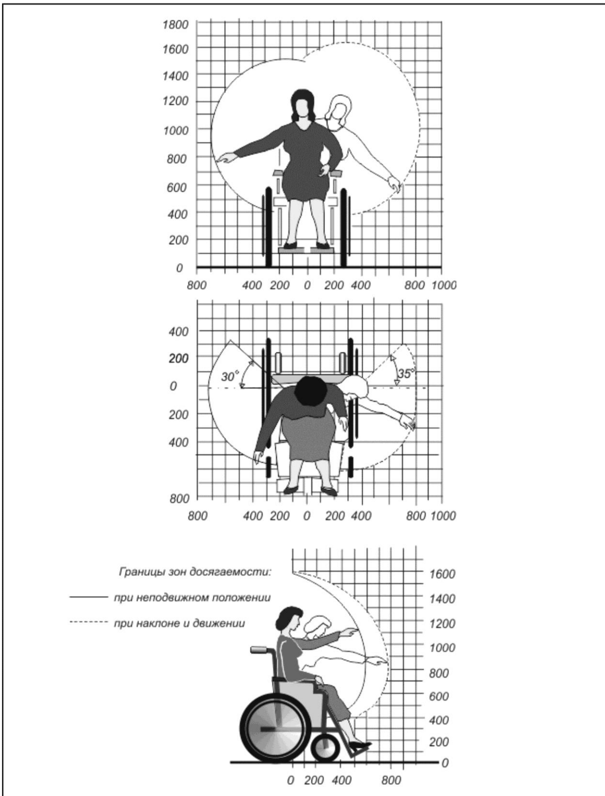
Рисунок Г.2 Зоны досягаемости инвалидов на кресле-коляске для женщин
