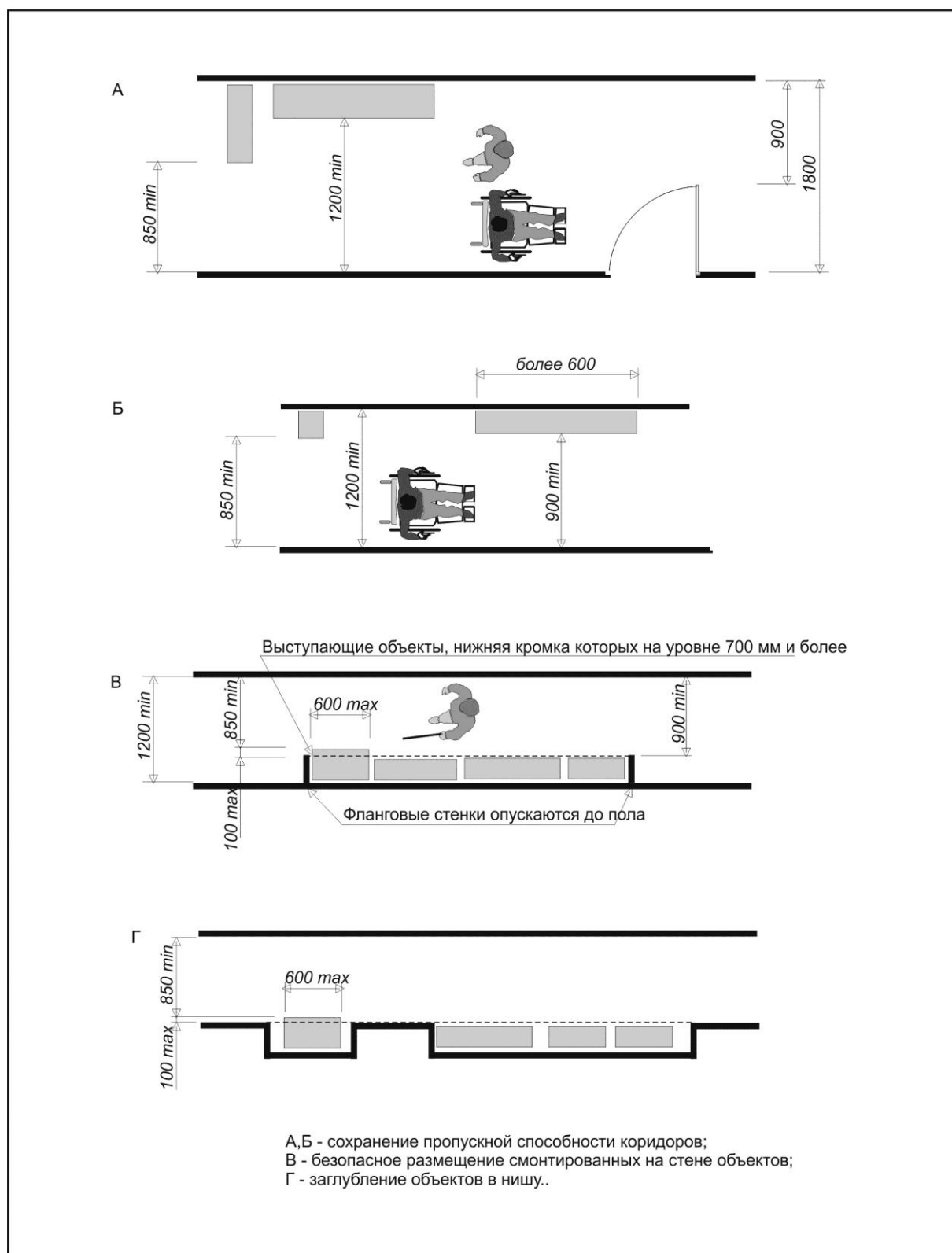
Рисунок В.10 Преграды в коридорах
