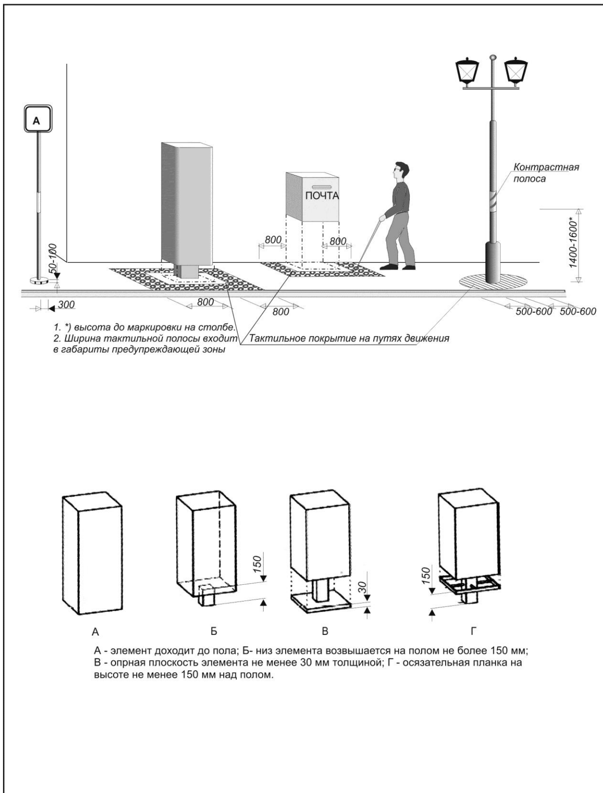
Рисунок В.4 Преграды на путях движения около зданий
