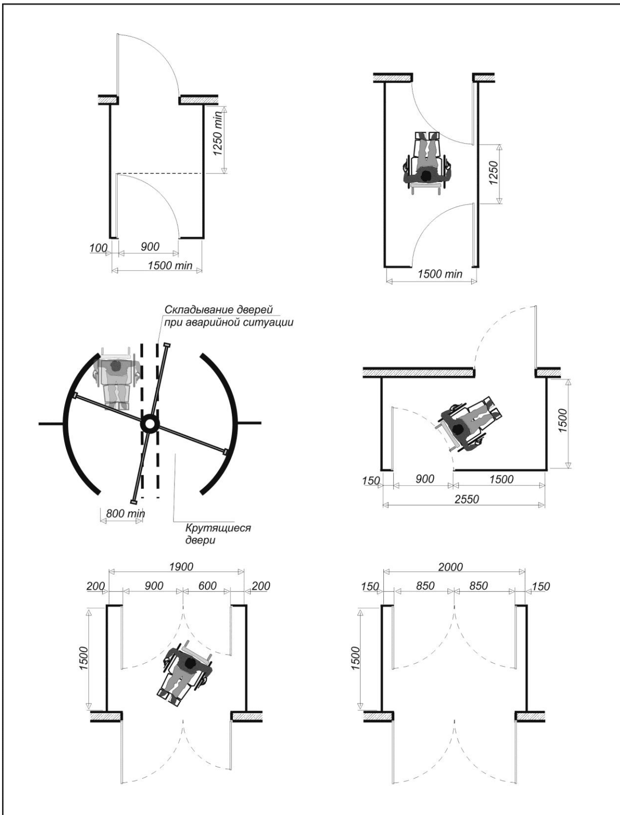
Рисунок В.15 Входные тамбуры
