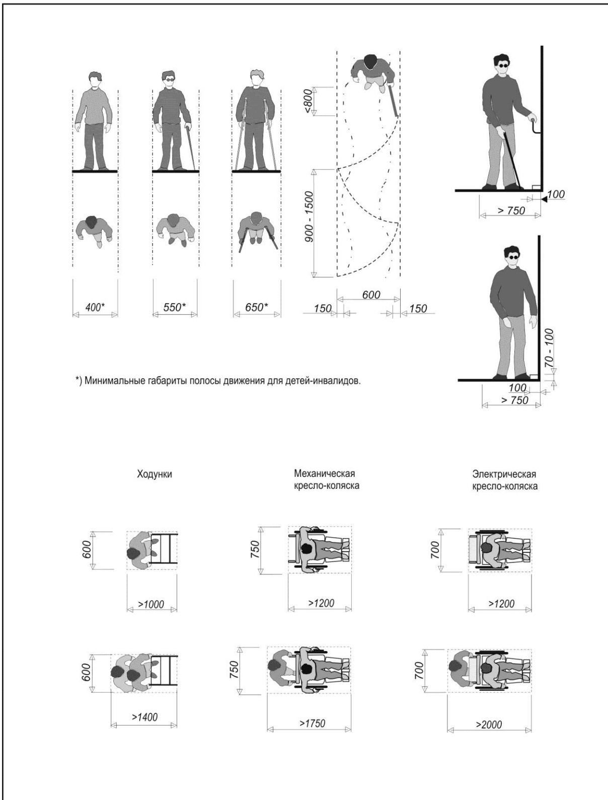
Рисунок В.11 Параметры зон движения инвалидов
