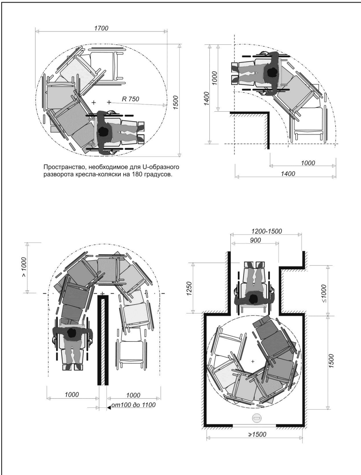
Рисунок В.9 Габариты поворотов и разворотов кресла-коляски
