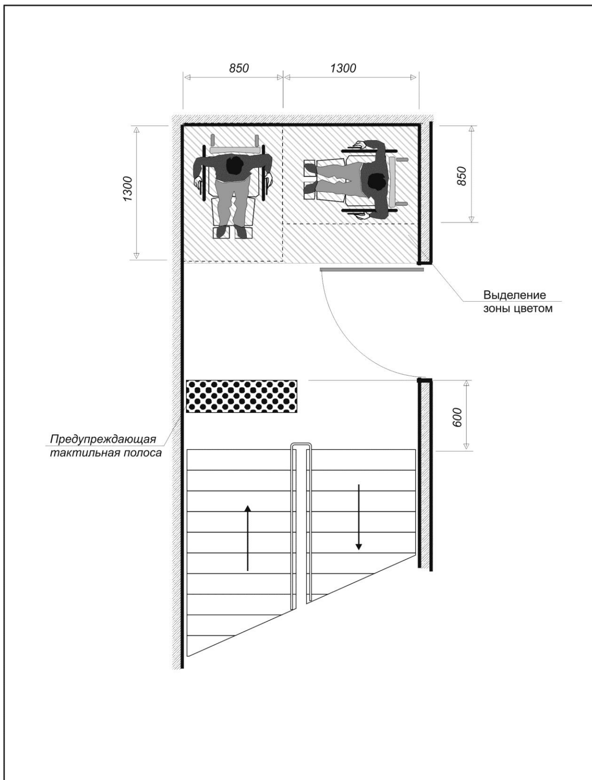
Рисунки В.20 Зона-накопитель для инвалидов на лестничной клетке при эвакуации
