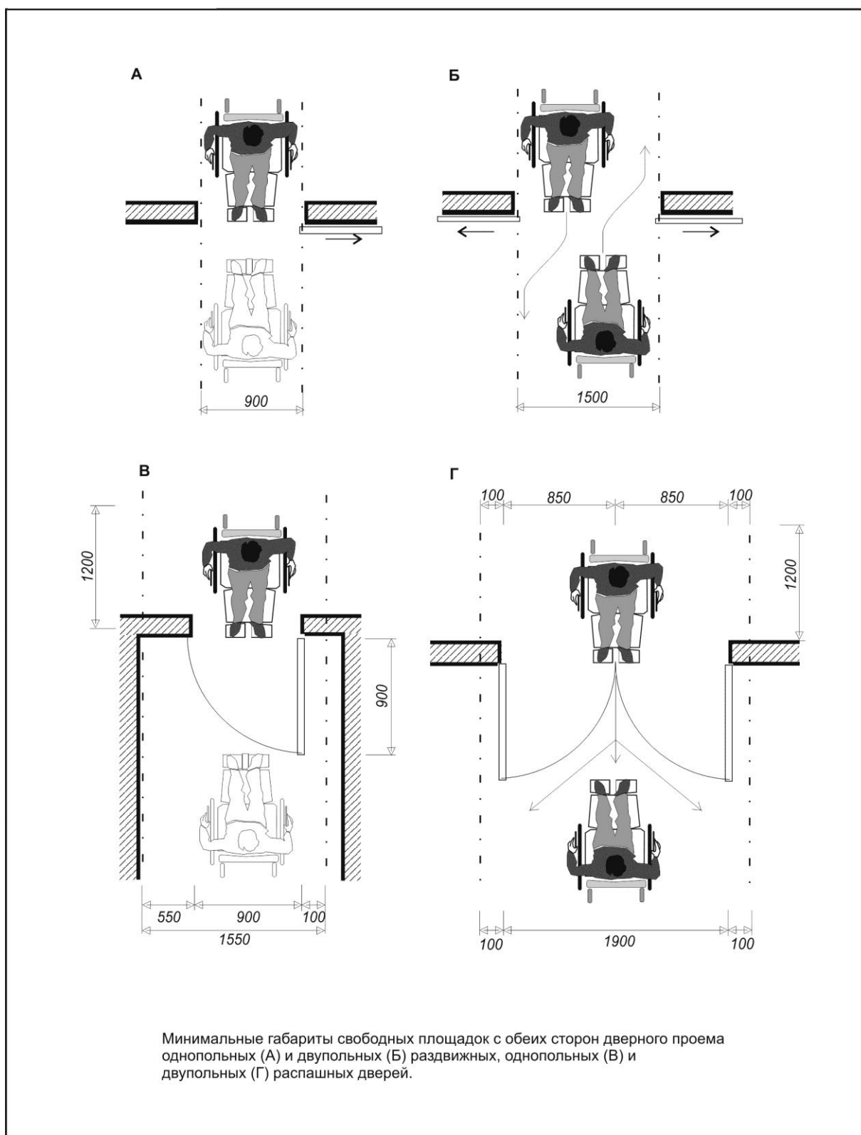
Рисунок В.12 Габариты площадок перед дверными проемами
