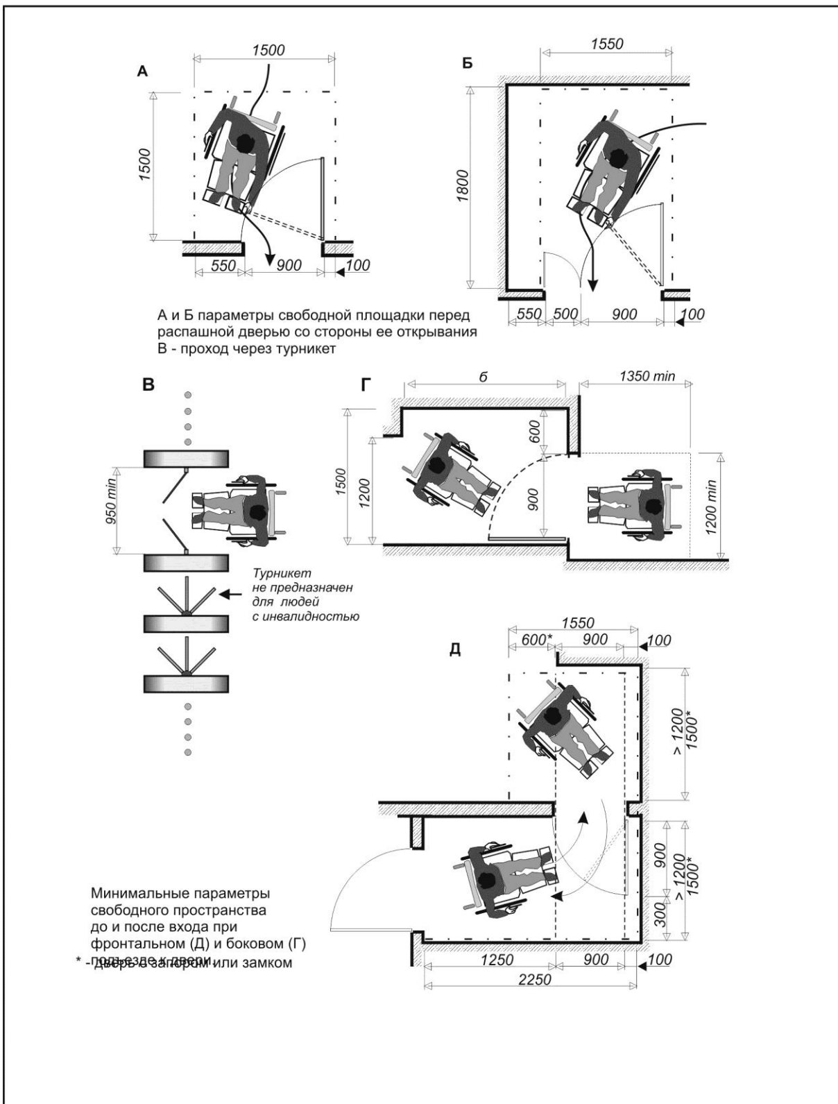
Рисунок В.14 Параметры входных площадок
