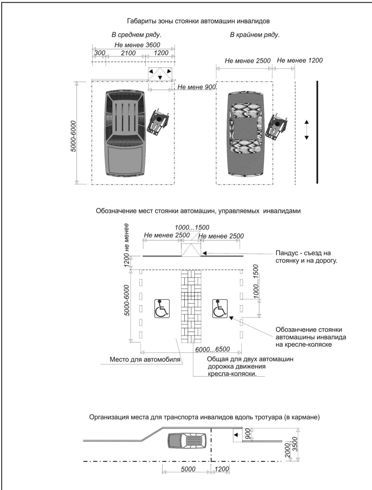
Рисунок В.7 Автостоянки
