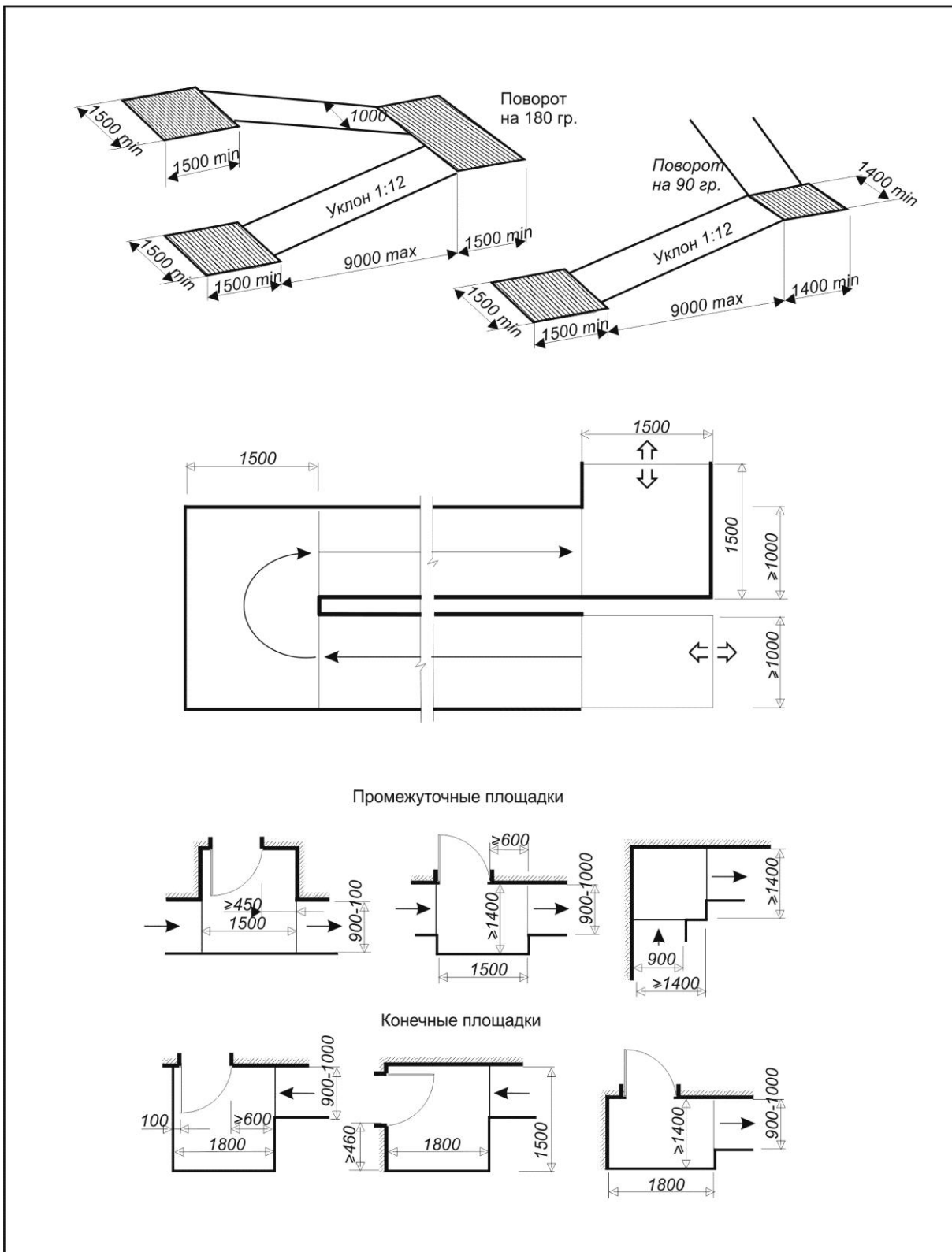
Рисунок В.21 Пандусы
