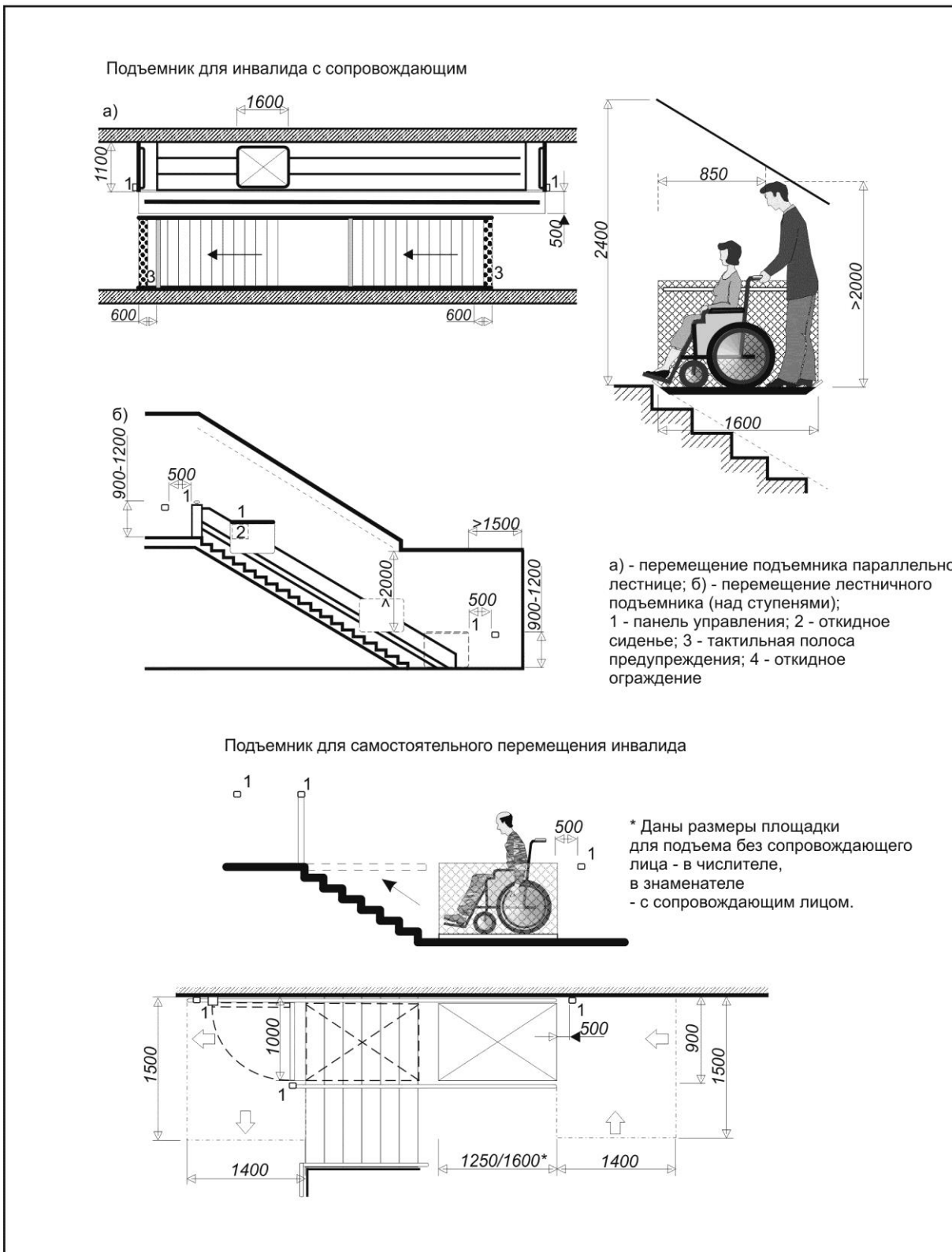
Рисунок В.25 Параметры наклонных подъемников
