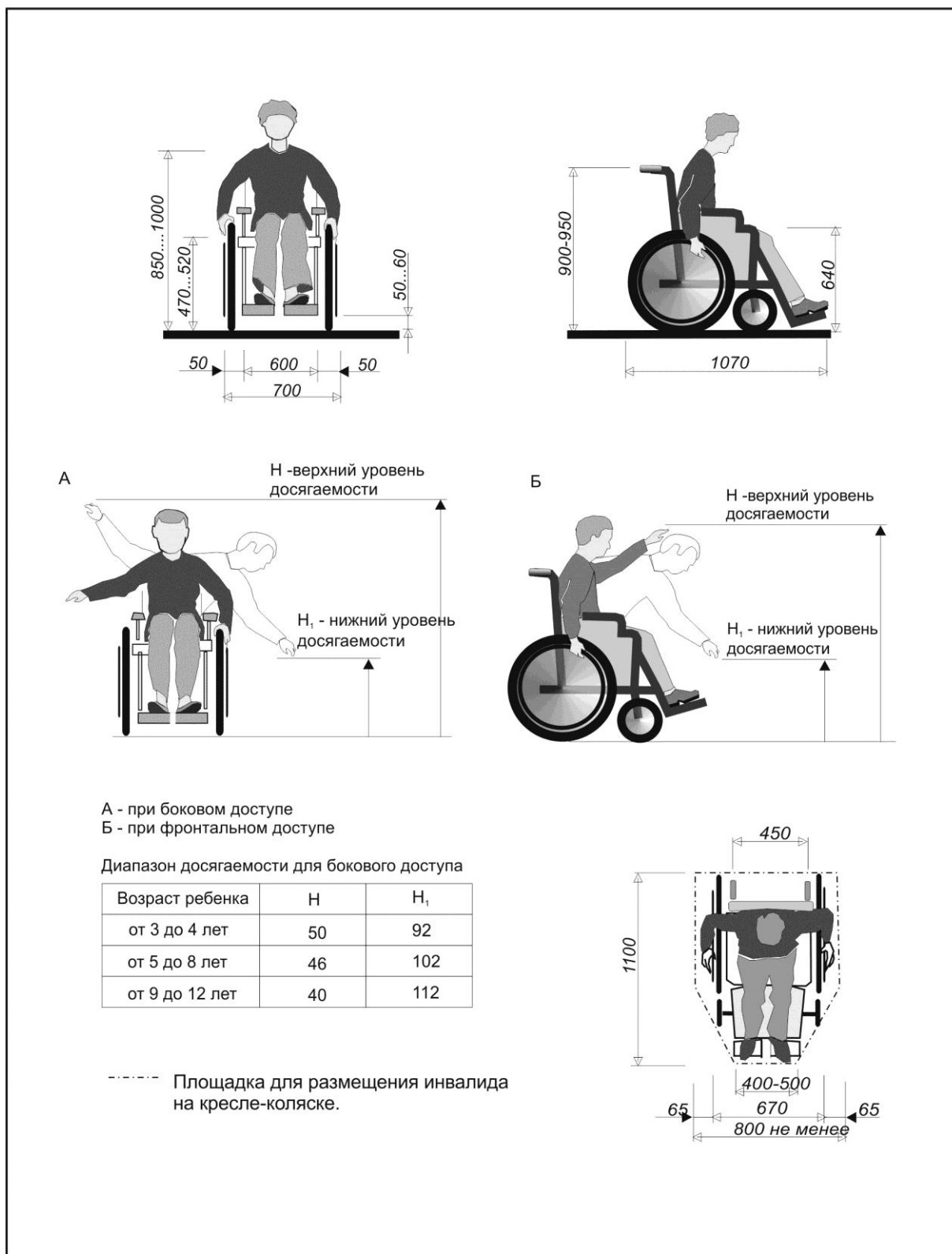
Рисунок В.2 Габариты кресла-коляски школьника и зоны досягаемости
